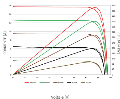
Curvas de corriente-voltaje y potencia-voltaje (500W)
